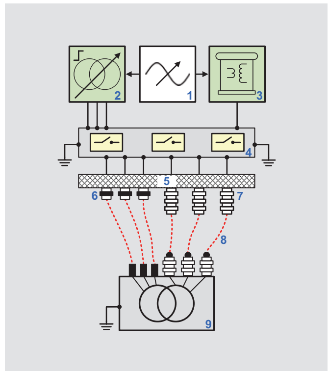
Figura 4 Dibujo esquemático del sistema de conmutación automática
