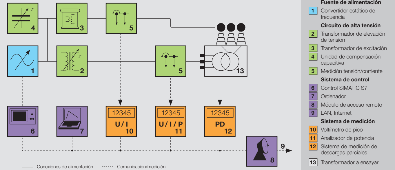
Fig. 3 Diagrama de bloques para el ensayo de transformadores en fábrica
